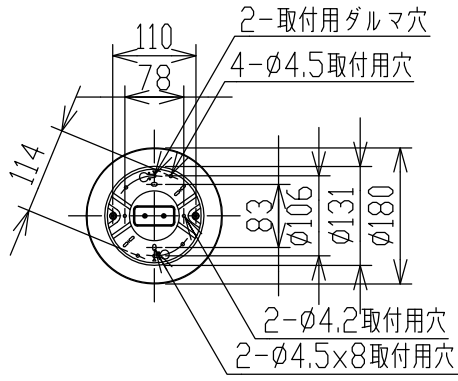
取付寸法(矢視①)
