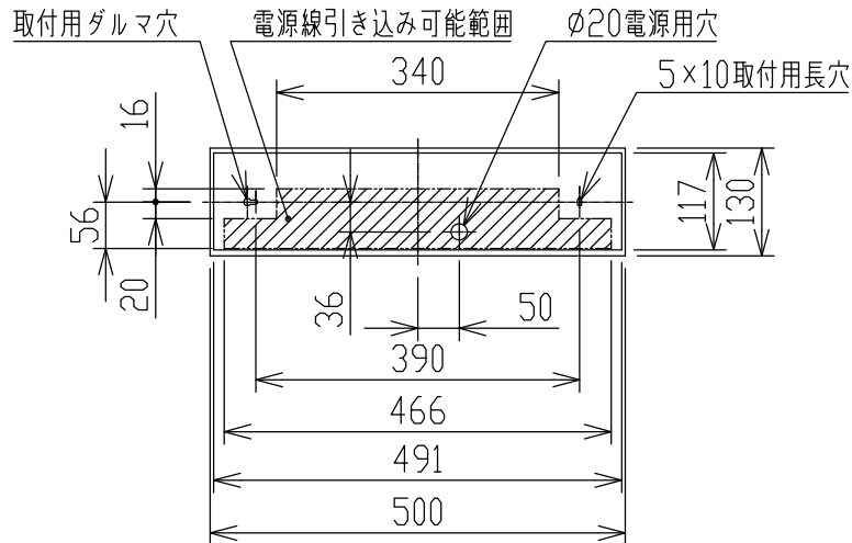
取付寸法(矢視①)
