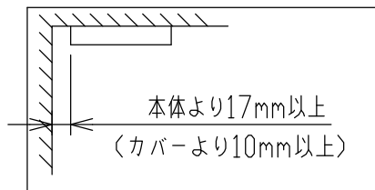
〈壁へ近接して取付する場合〉
