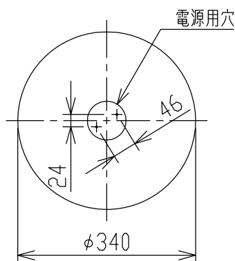
取付寸法(矢視 ②)
