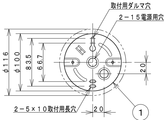
取付寸法 (矢視 a) (縮尺 1/4)
