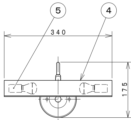
取付寸法 (矢視 a) (縮尺 1/4)
