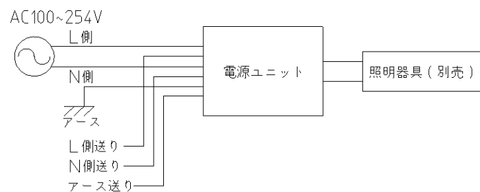
配線図
