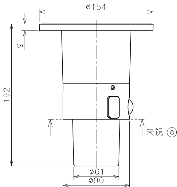
取付寸法（矢視 (a)）
