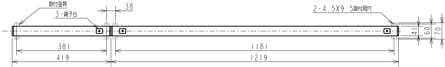
AL 43242L+AL 43257L 連結の場合
