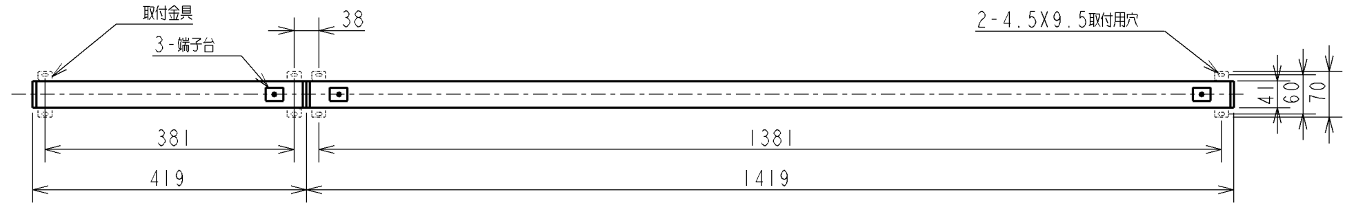
AL 43242L+AL 43262L 連結の場合
