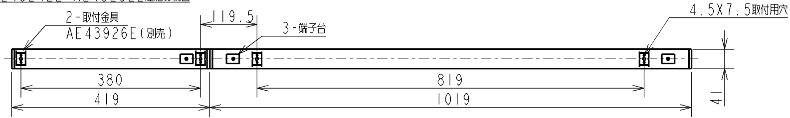
AL43242L+AL43252L 連結の場合
