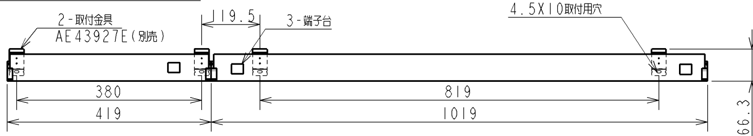
AL43242L+AL43257L 連結の場合
