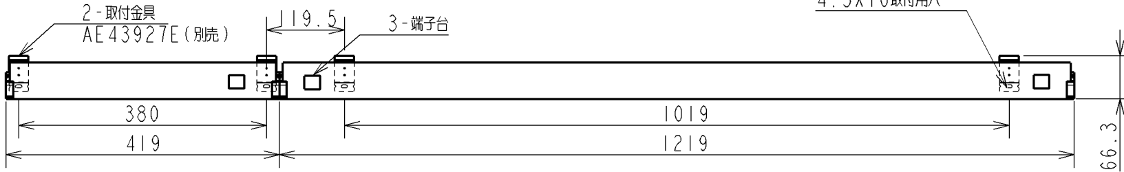
AL43242L+AL43262L 連結の場合
