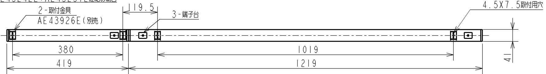
AL43242L+AL43262L 連結の場合
