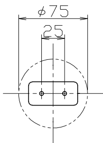
取付寸法（矢視 ㊶）
