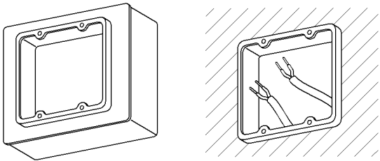
金属製Switchボックス2個用深形(カバー付):JIS C 8340
