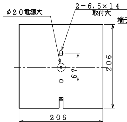
取付寸法（矢視 a）
