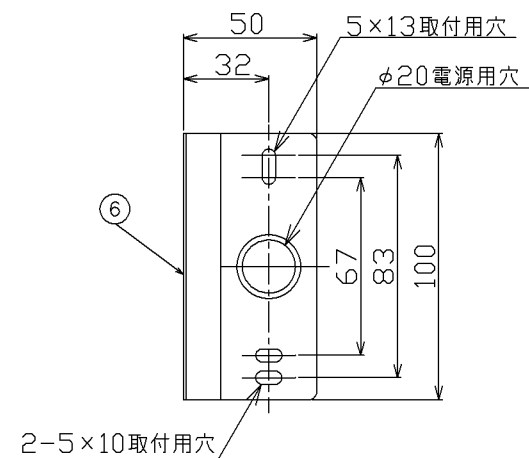
取付寸法（矢視④）
