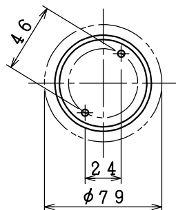
取付寸法(矢視⑧)
