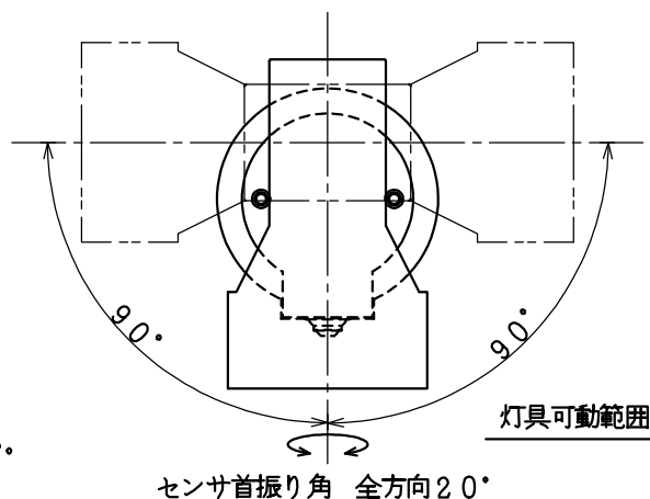
矢視⑨
