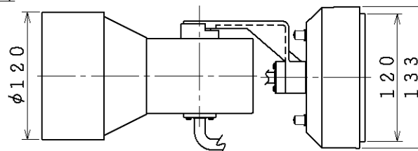
取付寸法（矢視③）
