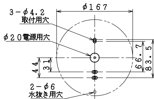
取付寸法 ( 矢視 ⑧ )
