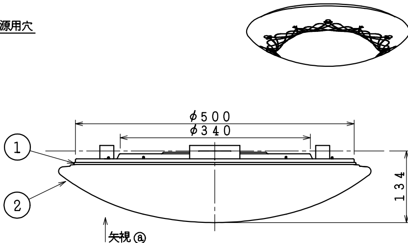
取付寸法(矢視 a)
