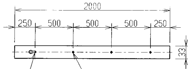
取付用ダルマ穴
