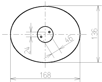
取付寸法 (矢視 a)
