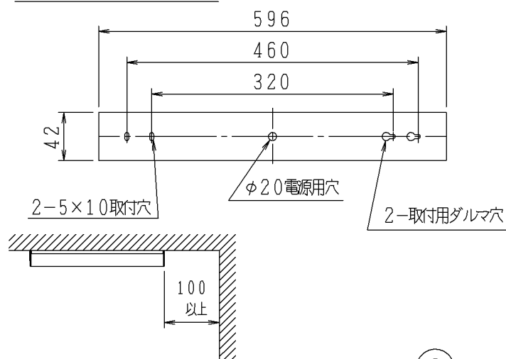
取付寸法（矢視 ②）
