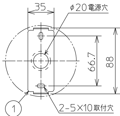
取付寸法 矢視a
