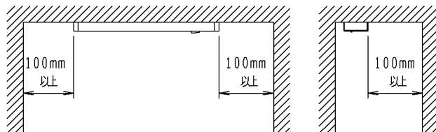
取付寸法 壁付の場合（矢視 ㊸）
