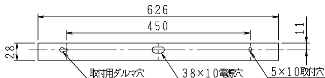
取付寸法 直付の場合（矢視 ㊹）
