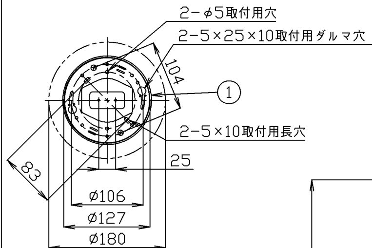
取付寸法 (③ 矢視)
