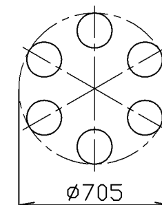
灯具配置図
