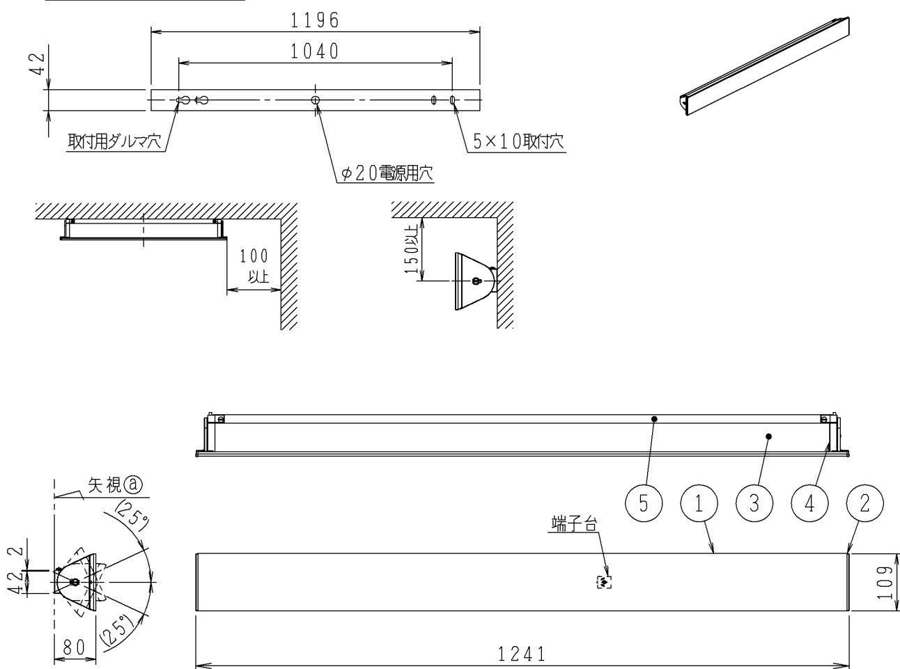
取付寸法（矢視 ㊸）
