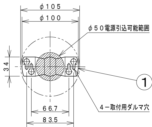
取付寸法（矢視 a） （縮尺 1/4）
