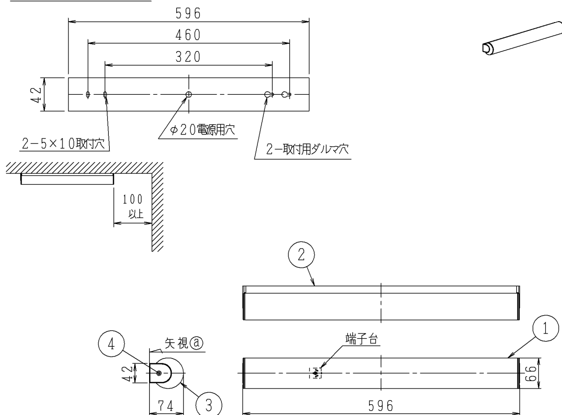
取付寸法（矢視 ①）
