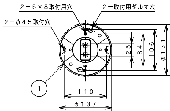
取付寸法（矢視 a）
