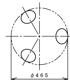
灯具配置図
