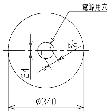
取付寸法(矢視 ㊸)
