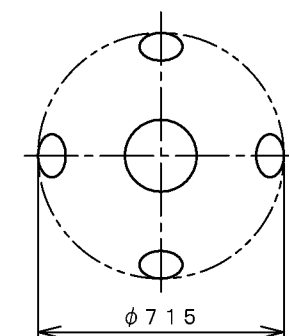
器具配置図
