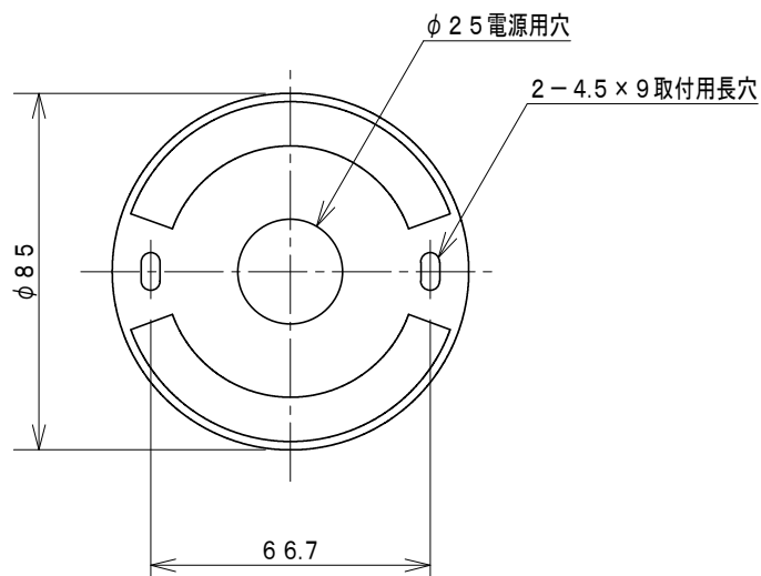
取付寸法 (矢視 a)
