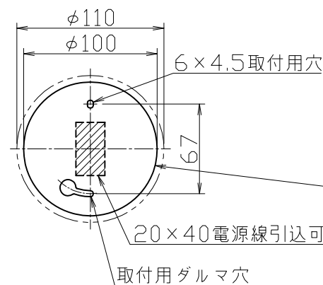
取付寸法（矢視 ㉑）
