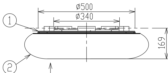
矢視 ①
