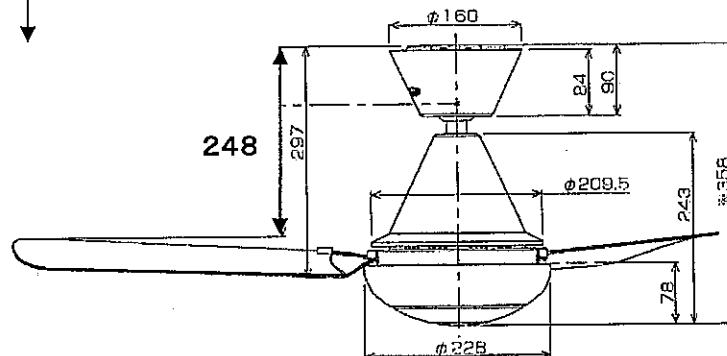
矢視①
