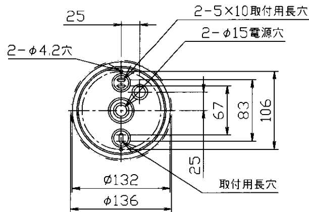
取付寸法（矢視 ①）
