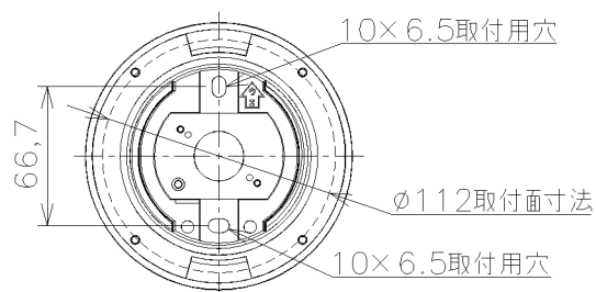
取付寸法（矢視 ①）
