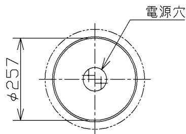
取付寸法 (矢視㊸)
