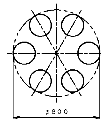
灯具配置図
