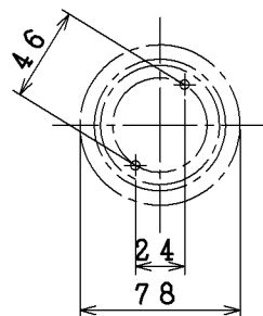
取付寸法(矢視⑨)
