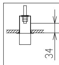
ボルト引込しろ
