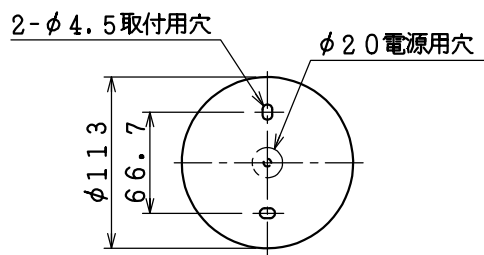
取付寸法(矢視 ⑧)
