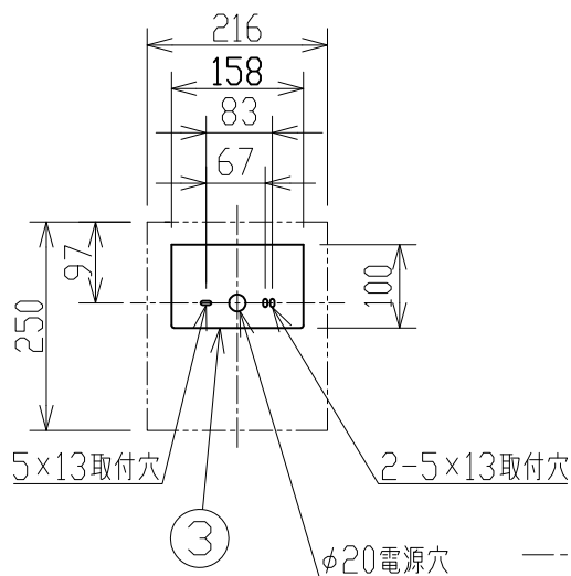
取付寸法(矢視 a) (縮尺1/10)
