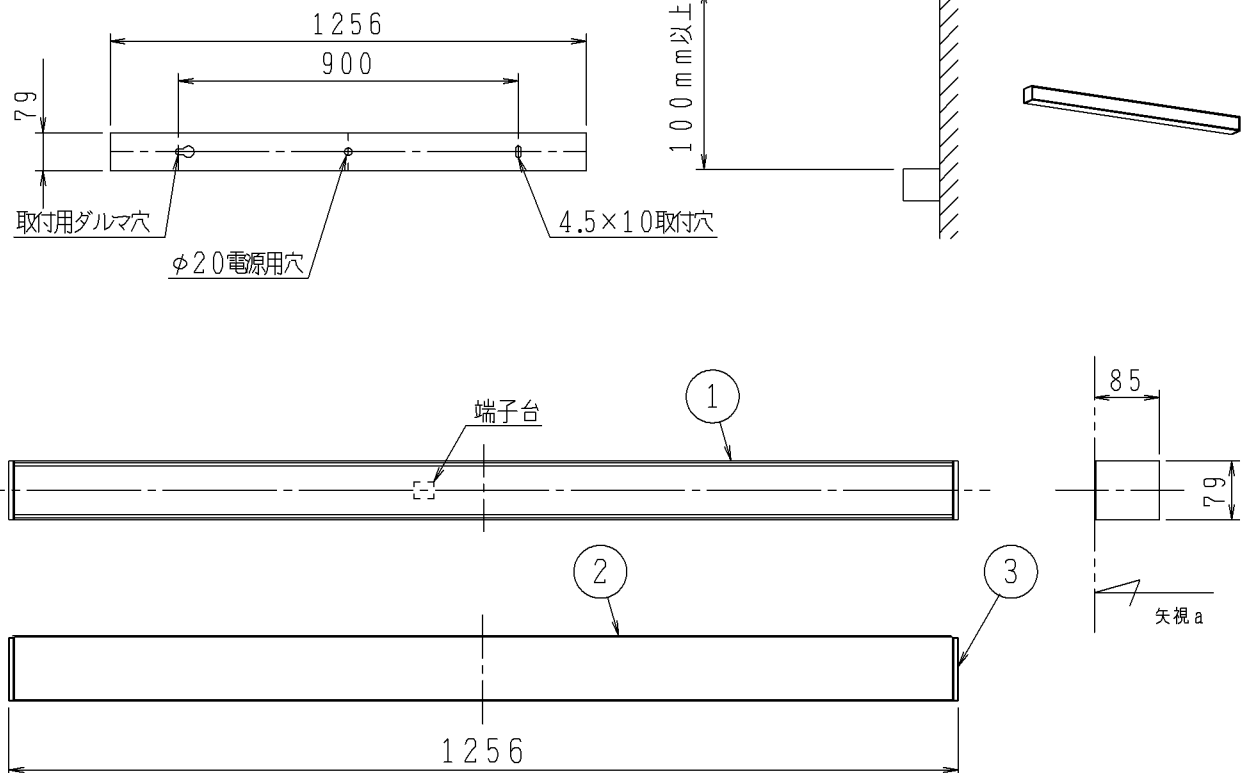
取付寸法（矢視 ①）
