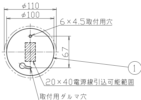
取付寸法（矢視 ①）
