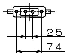
取付寸法（矢視 ㊸）
