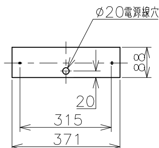
天井取付寸法（矢視 ㊹）
