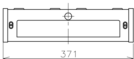
壁取付寸法（矢視 ㊸）
