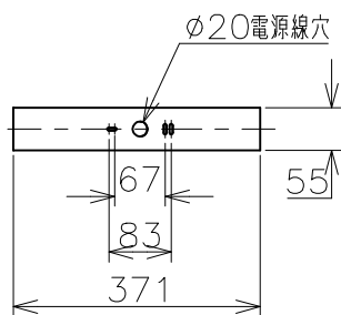
壁取付寸法（矢視 ㊸）
