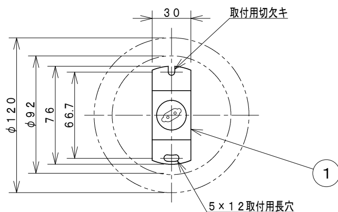
取付寸法 (矢視 a)
