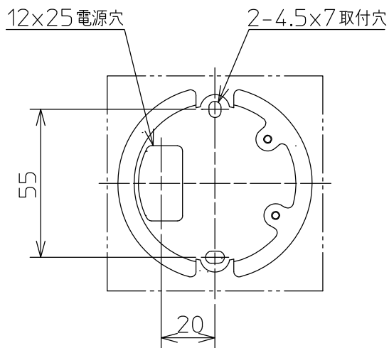
取付寸法 矢視a
