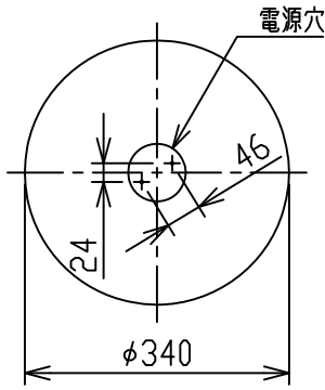
取付寸法(矢視 ㊸)
