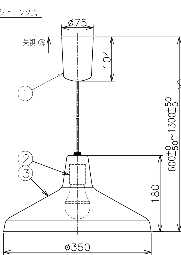
取付寸法 (矢視 @)
