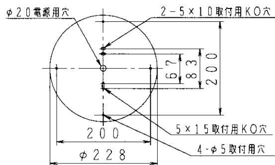
取付寸法（矢視 ①）
