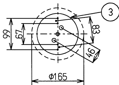
取付寸法 (矢視 α)
